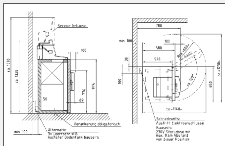
CASHDROP ecco stand alone nach Zeichnung A-ELS 200-000-47-3-00
